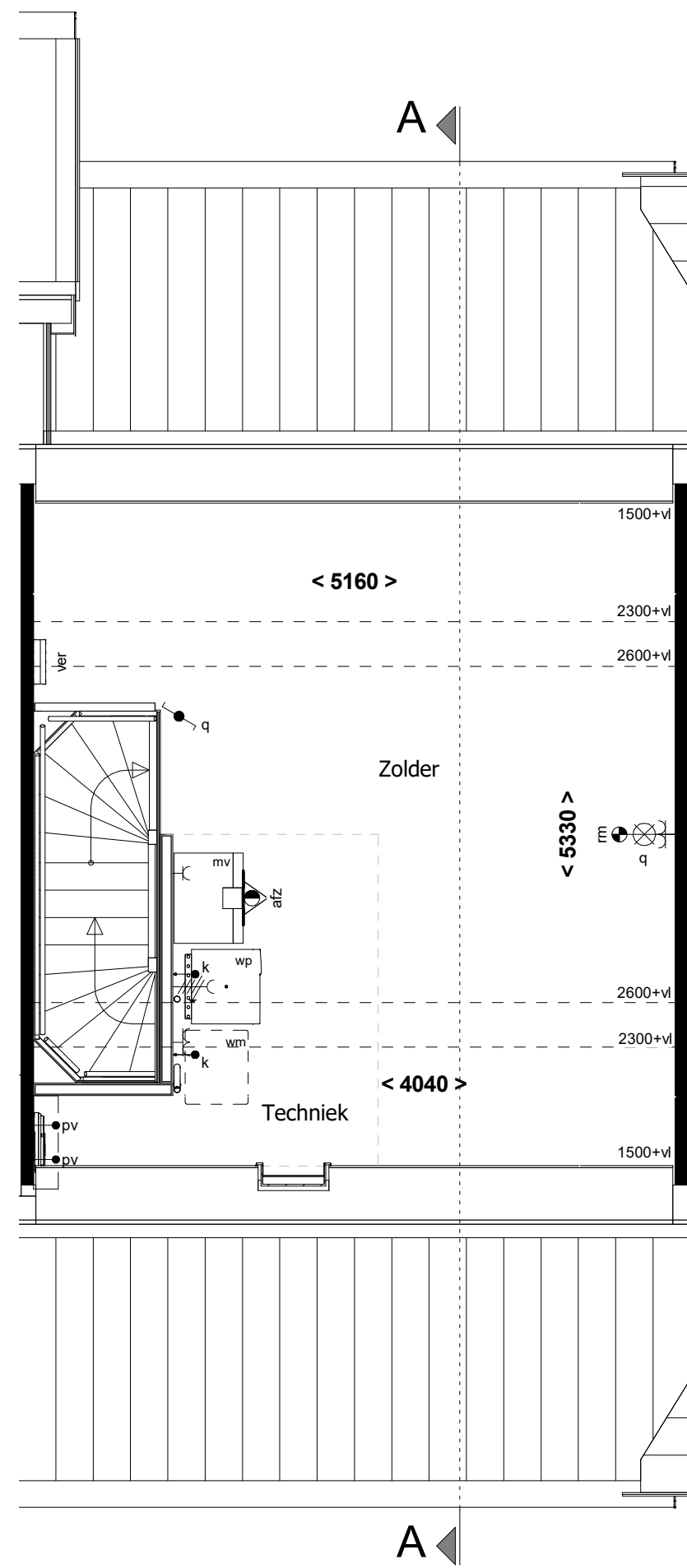
2e verdieping 1 : 50
