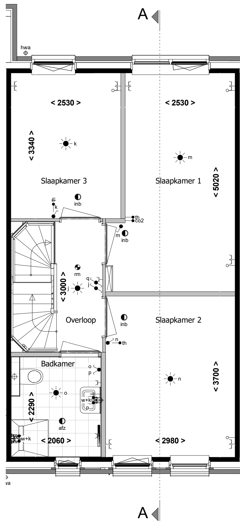
1e verdieping 1 : 50
