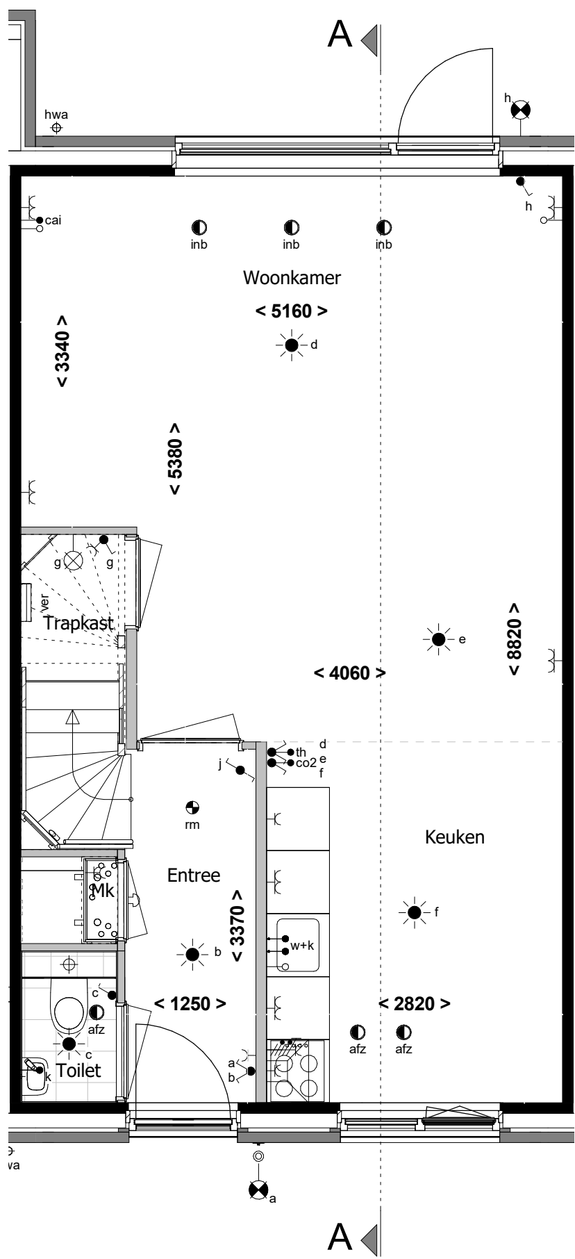
Begane grond 1 : 50
