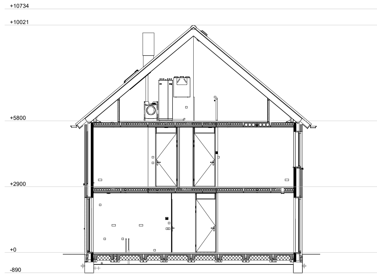
Doorsnede A-A 1 : 100
