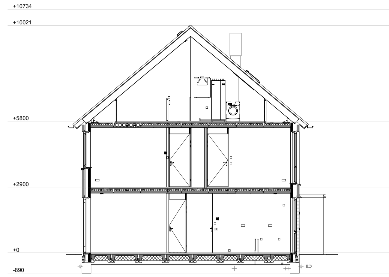
Doorsnede A-A 1 : 100
