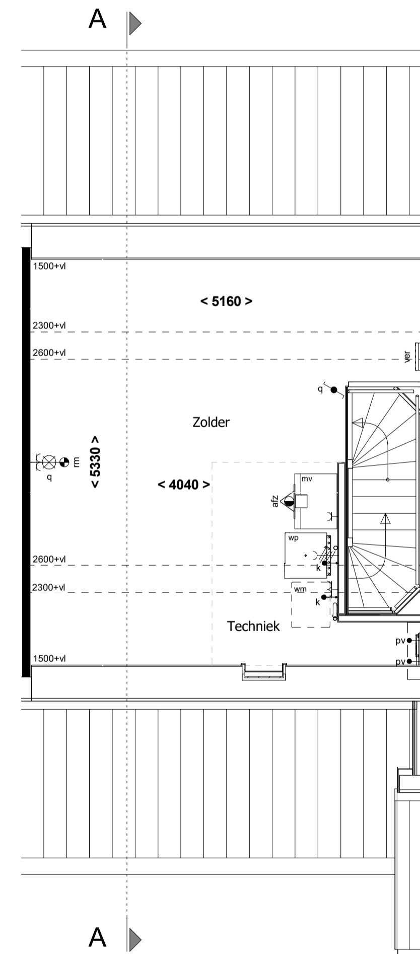
2e verdieping 1 : 50
