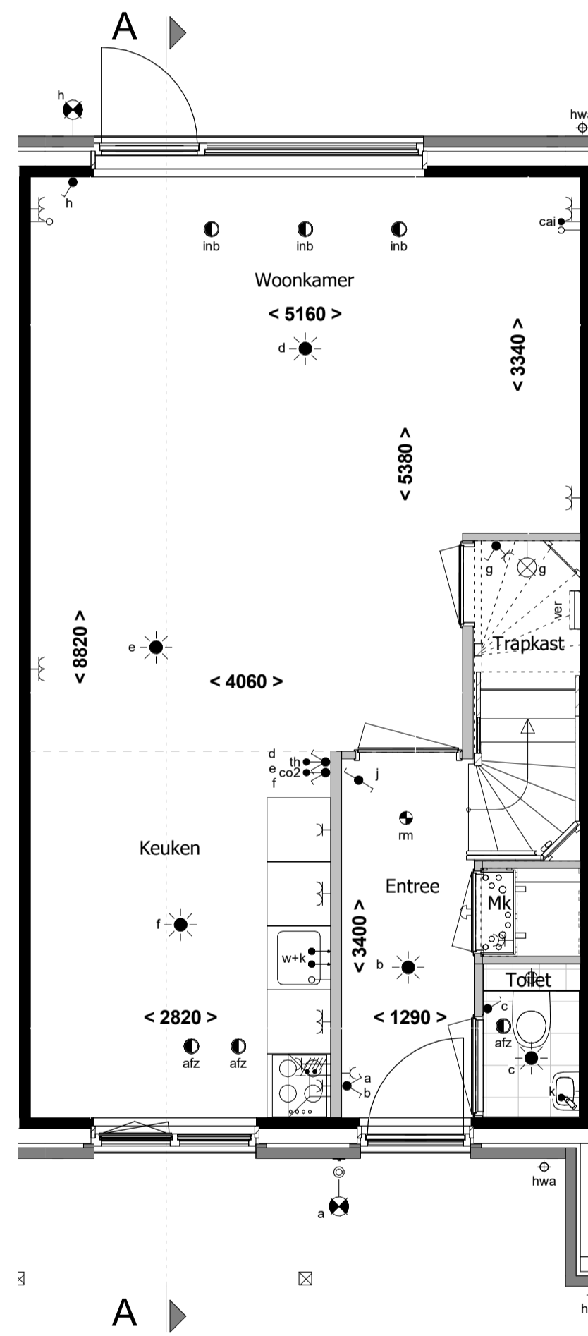
Begane grond 1 : 50
