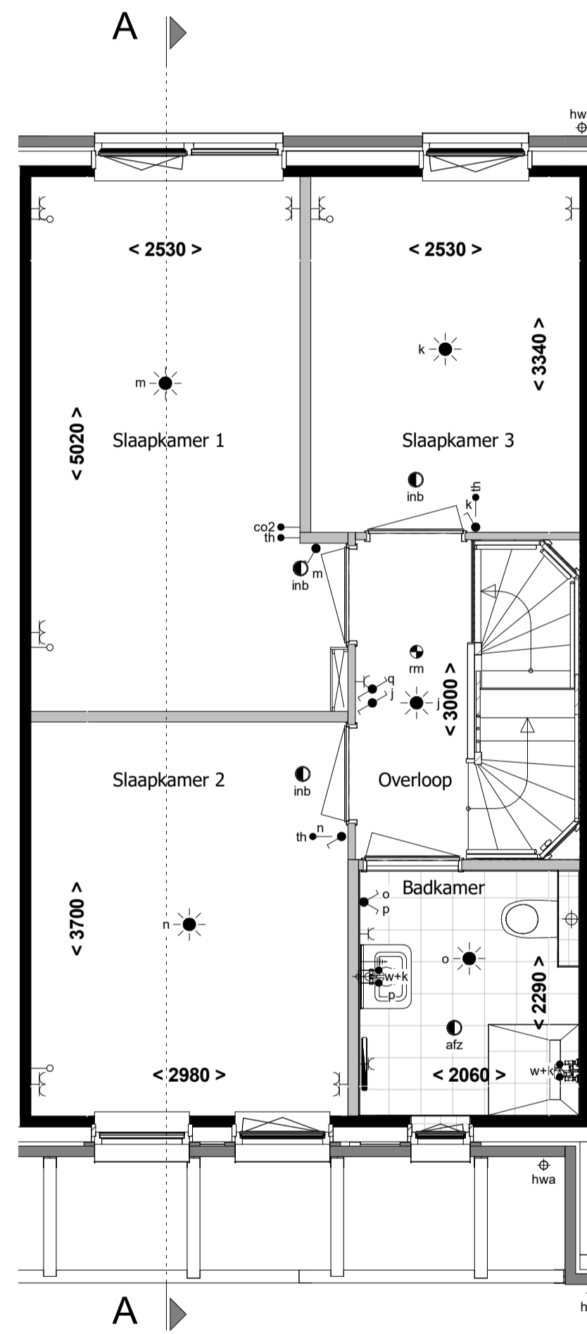
1e verdieping 1 : 50
