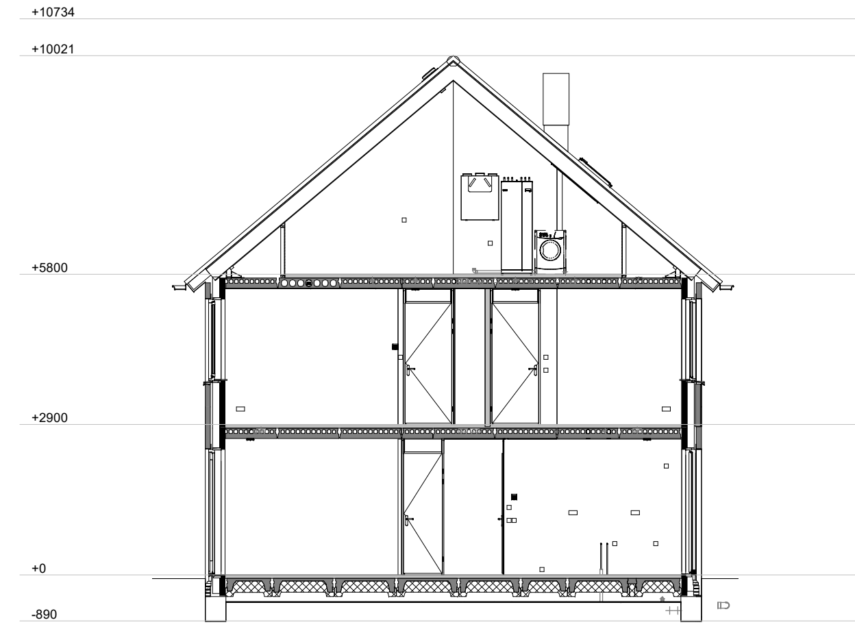
Doorsnede A-A 1 : 100
