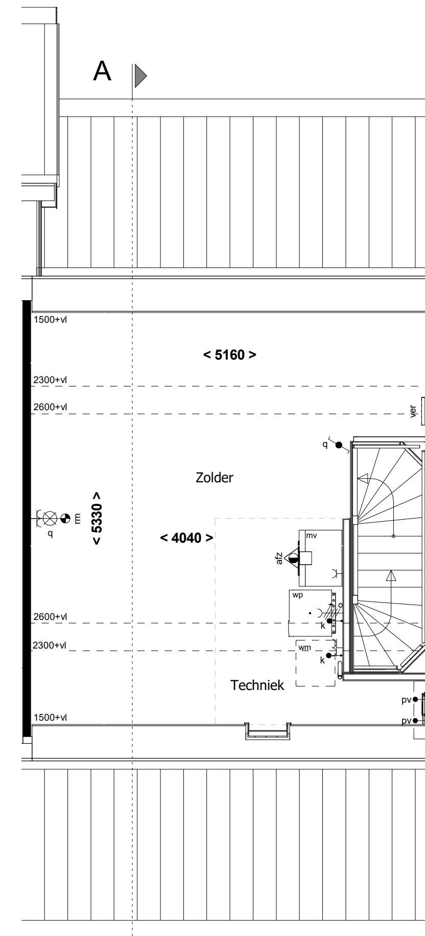
2e verdieping 1 : 50
