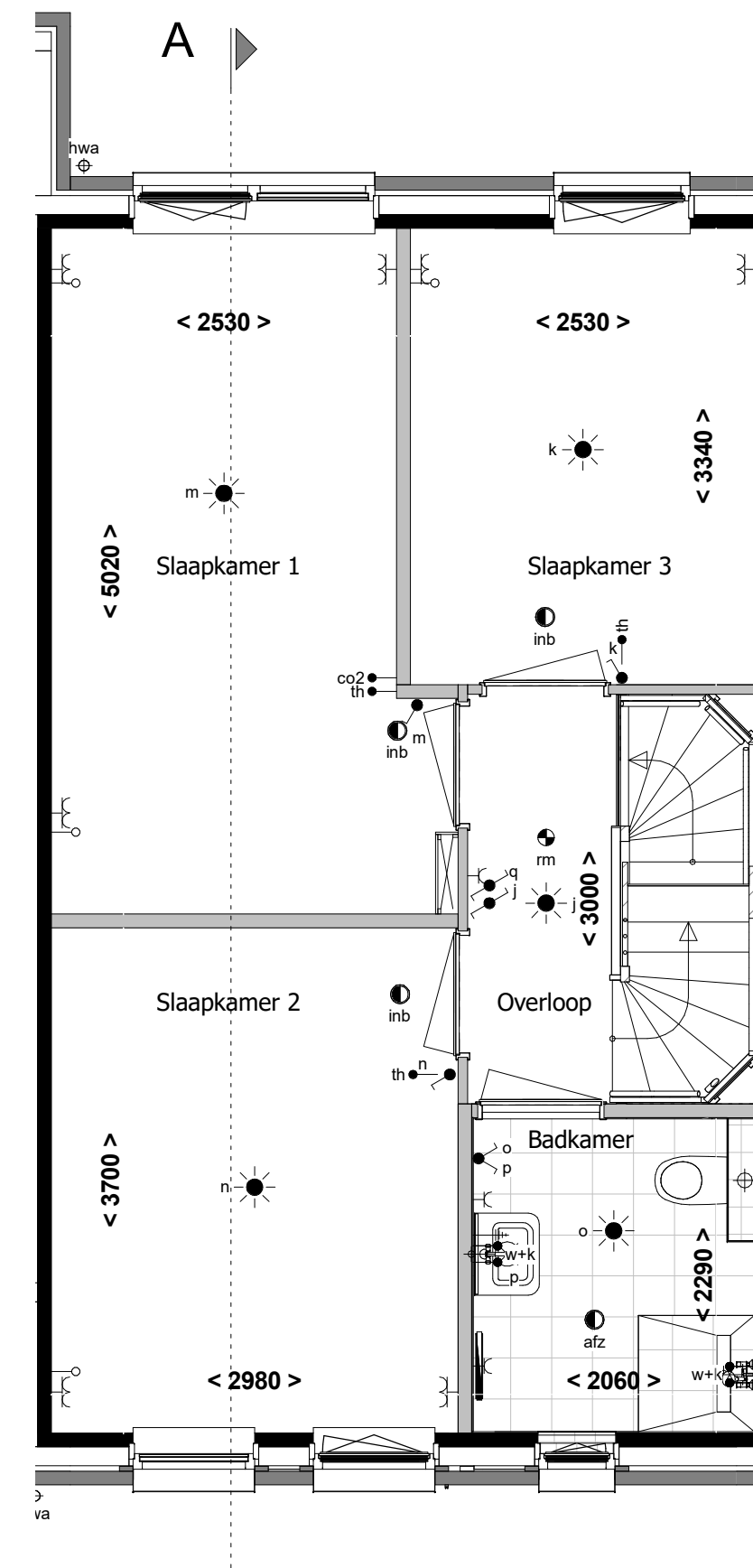
1e verdieping 1 : 50
