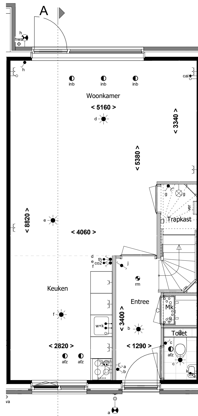
Begane grond 1 : 50
