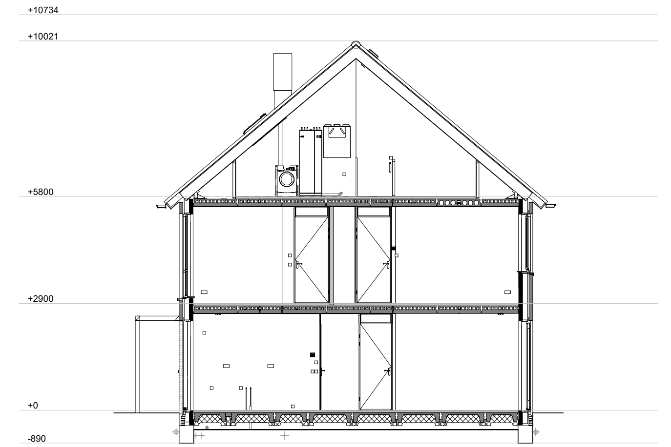
Doorsnede A-A 1 : 100
