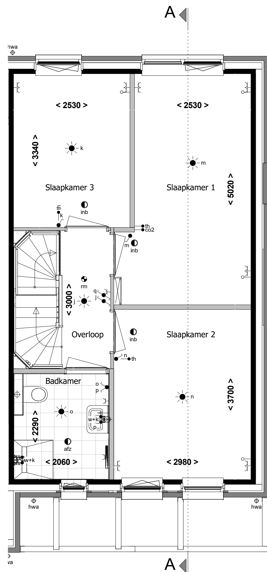
1e verdieping 1 : 50
