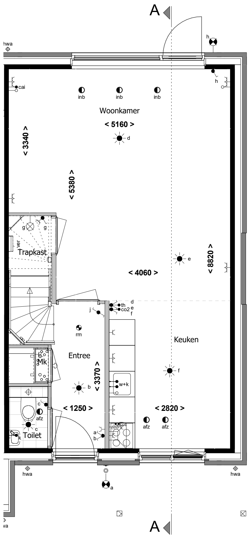
Begane grond 1 : 50
