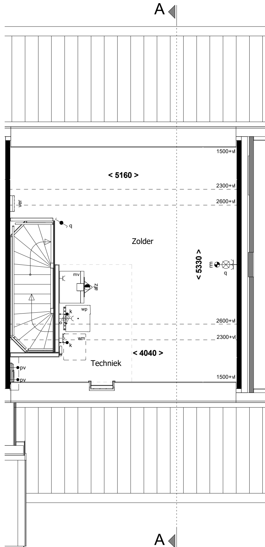
2e verdieping 1 : 50
