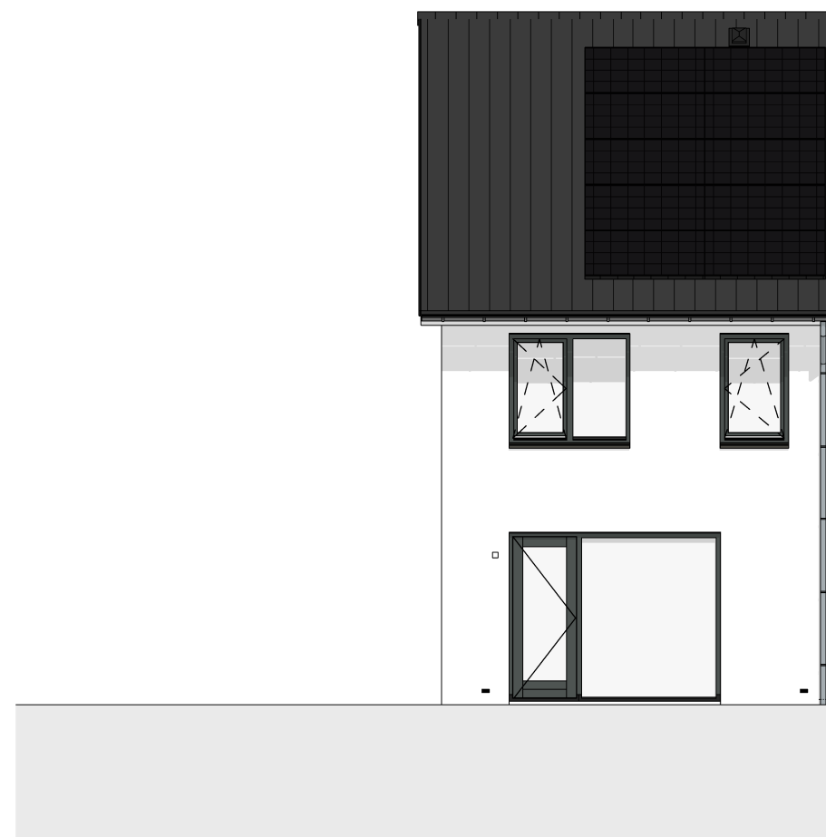
Achtergevel 1 : 100
