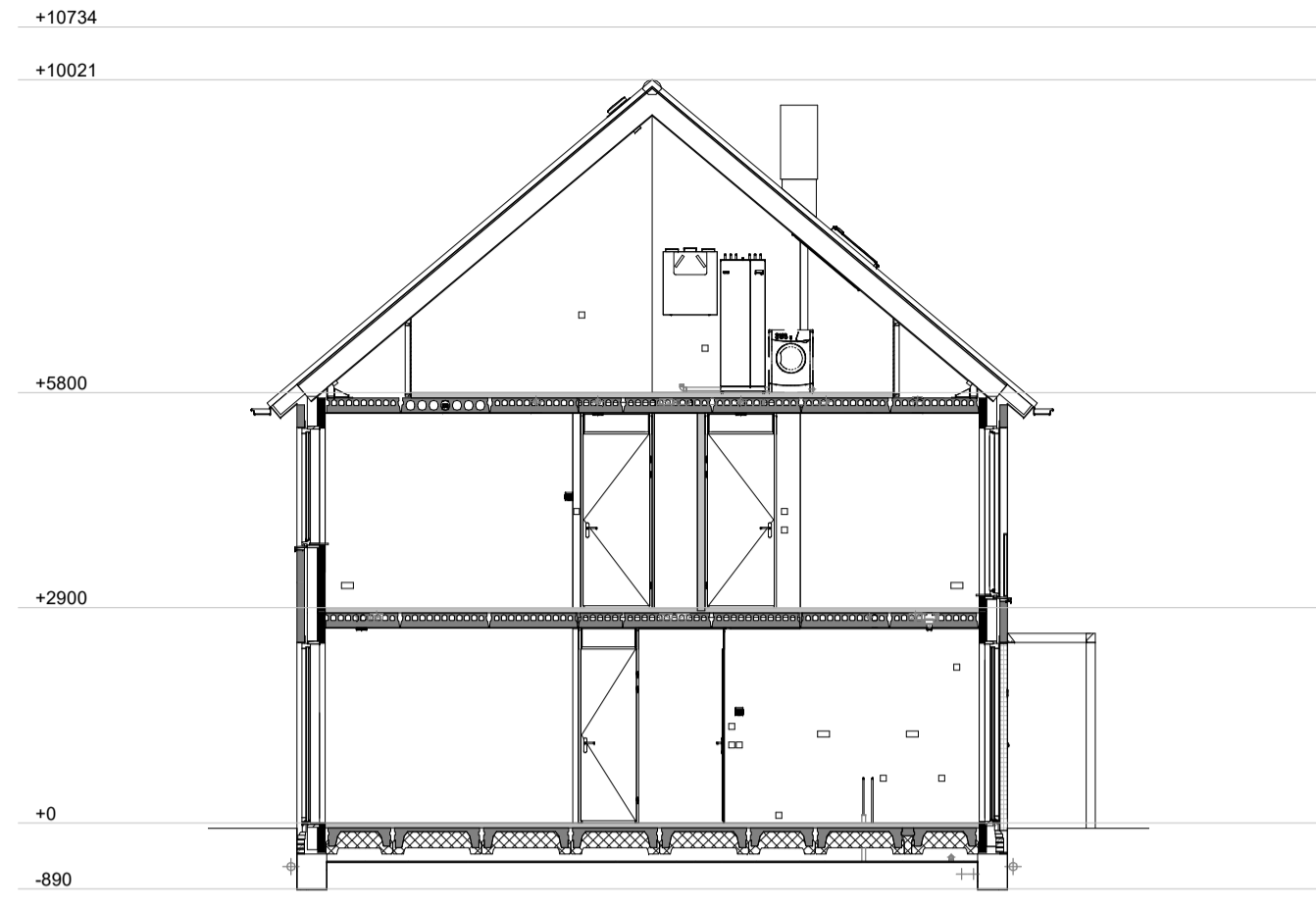
Doorsnede A-A 1 : 100
