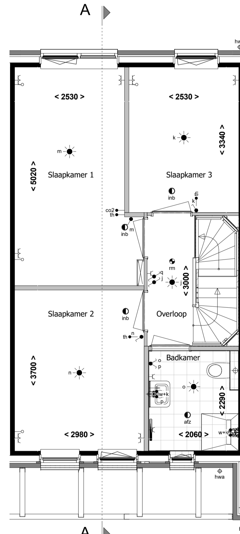
1e verdieping 1 : 50
