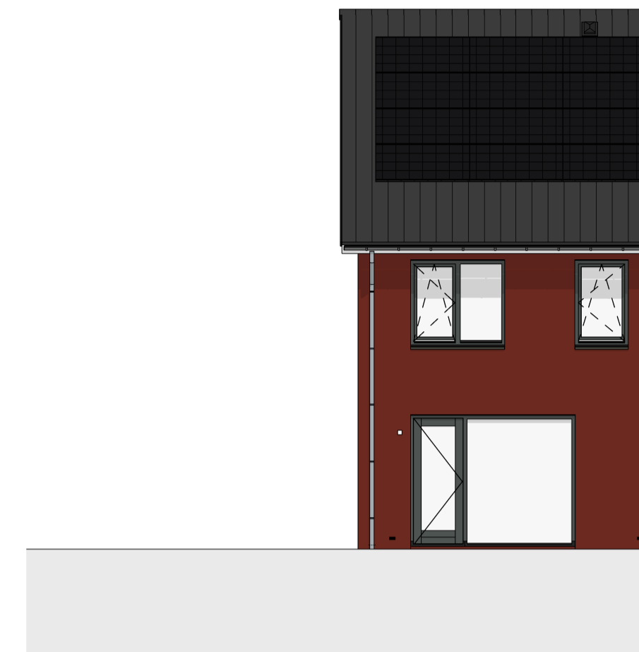
Achtergevel 1 : 100
