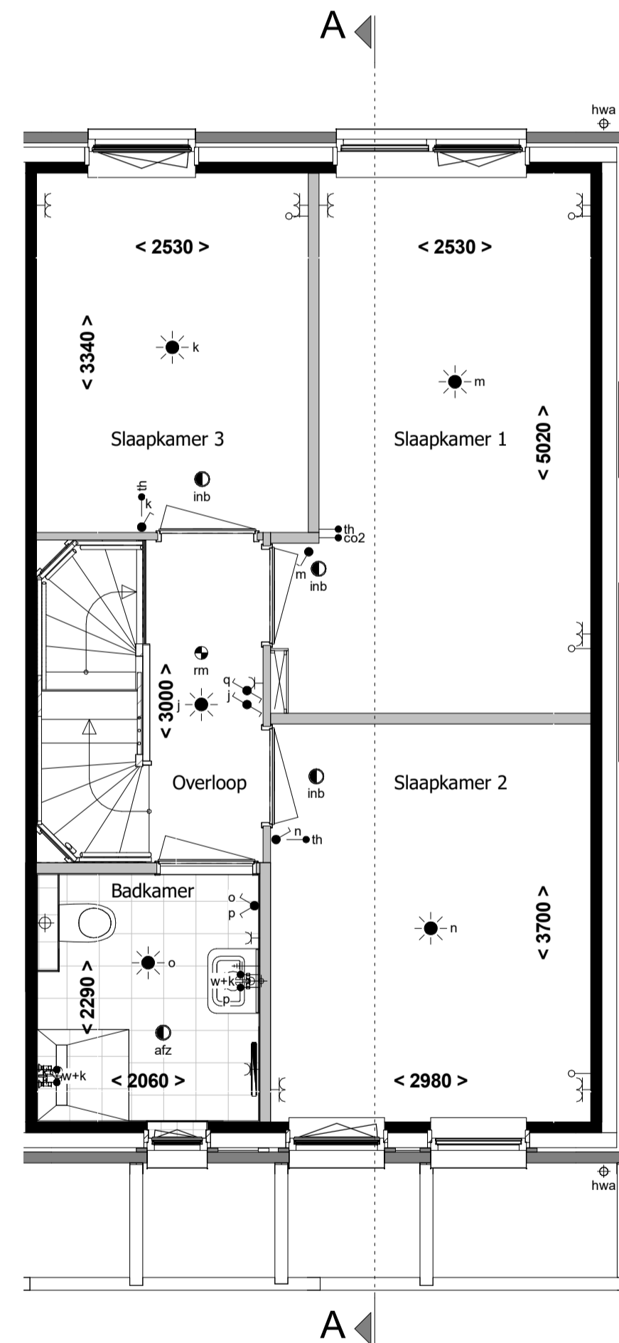
1e verdieping 1 : 50
