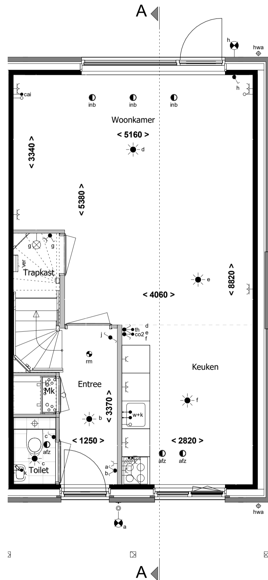
Begane grond 1 : 50
