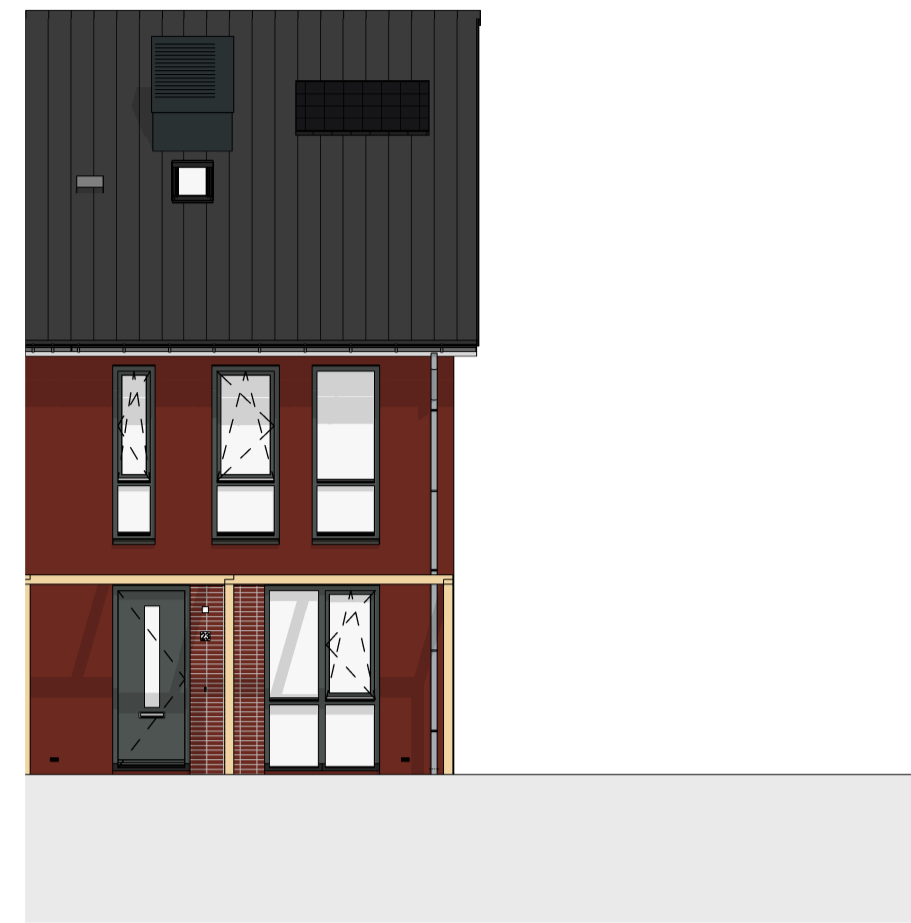
Voorgevel 1 : 100
