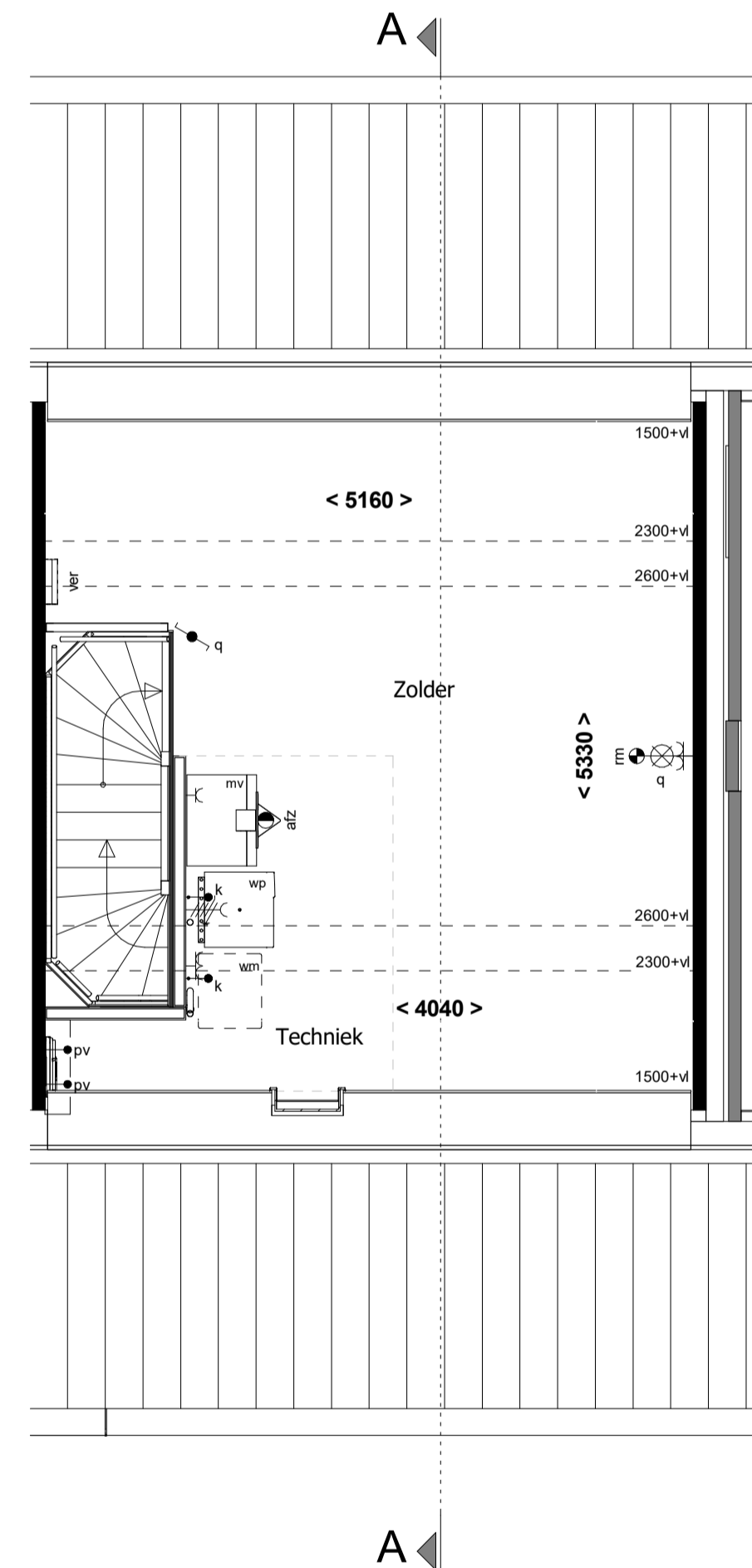
2e verdieping 1 : 50
