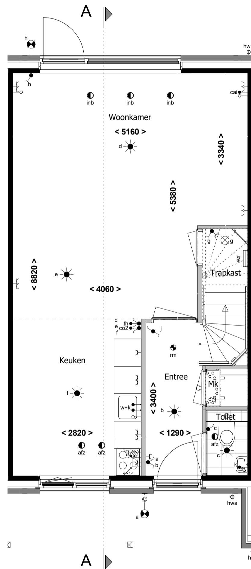
Begane grond 1 : 50
