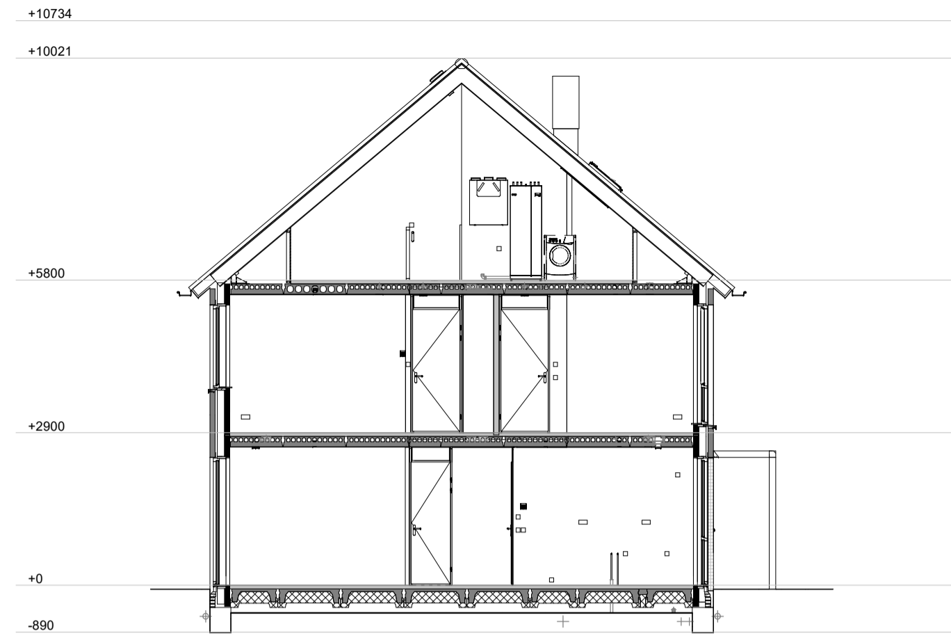
Doorsnede A-A 1 : 100
