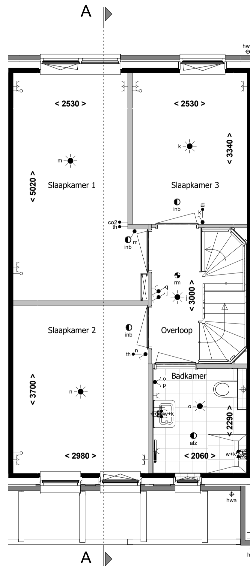
1e verdieping 1 : 50
