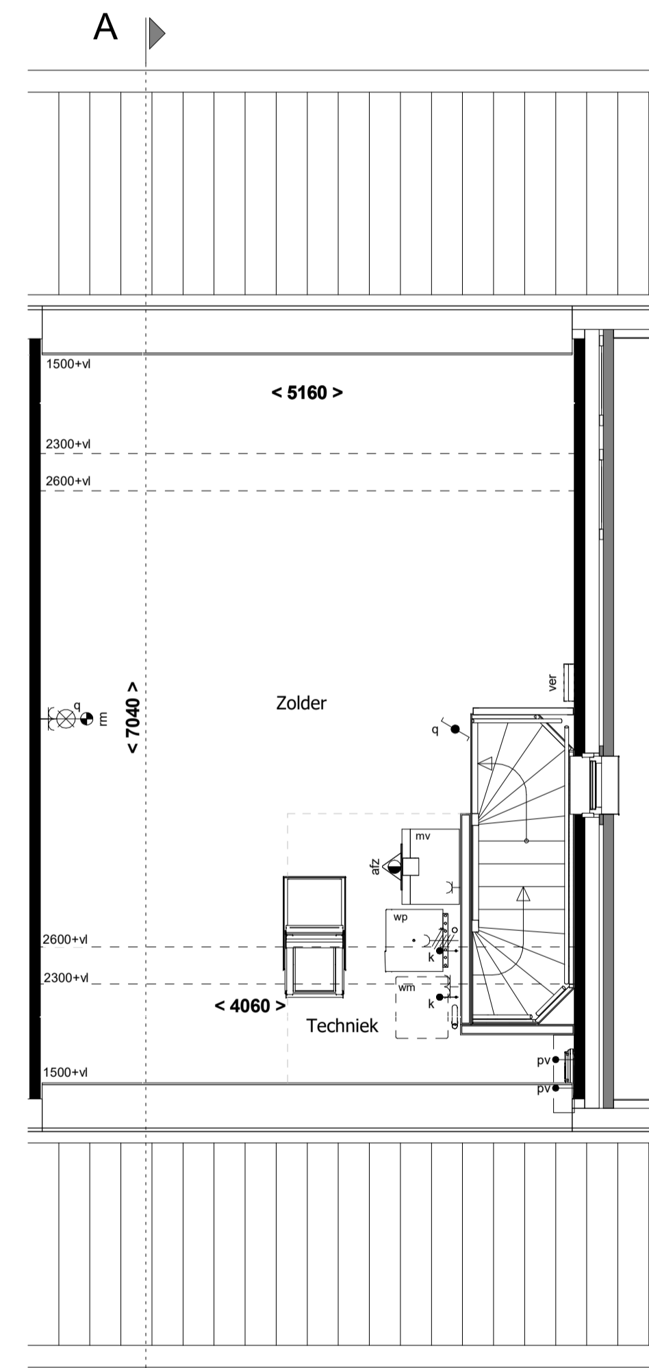
2e verdieping 1 : 50
