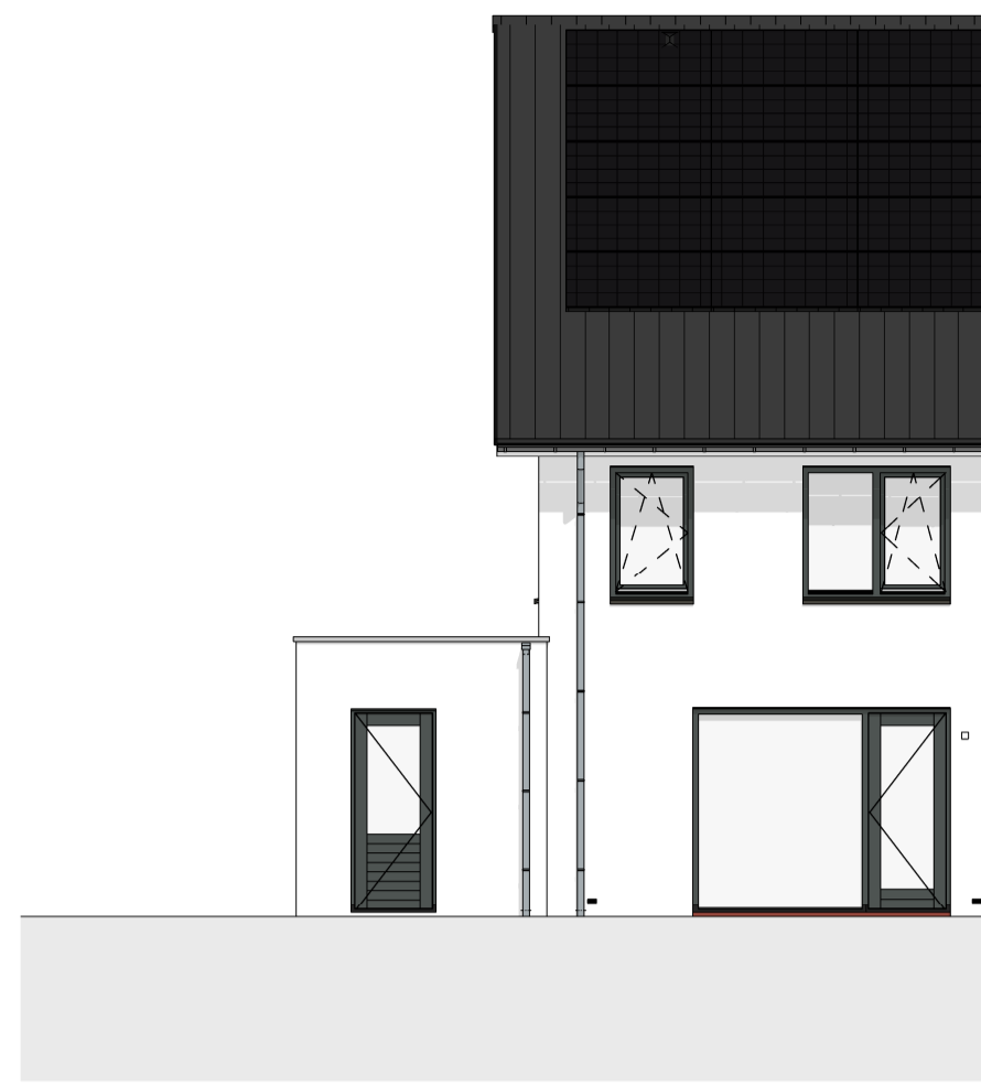
Achtergevel 1 : 100
