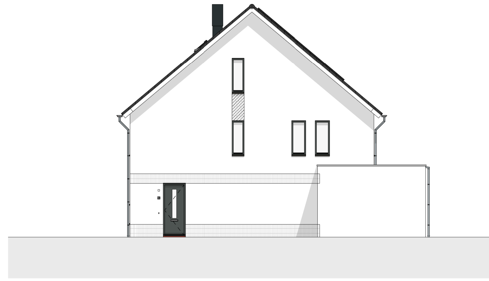
Rechter zijgevel 1 : 100
