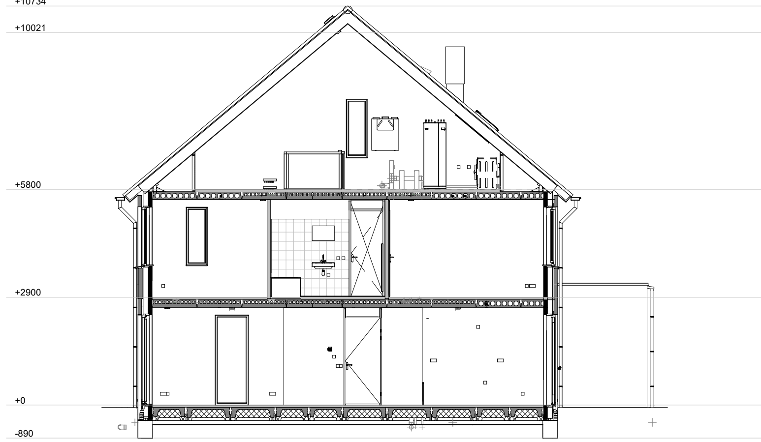
Doorsnede A-A 1 : 100
