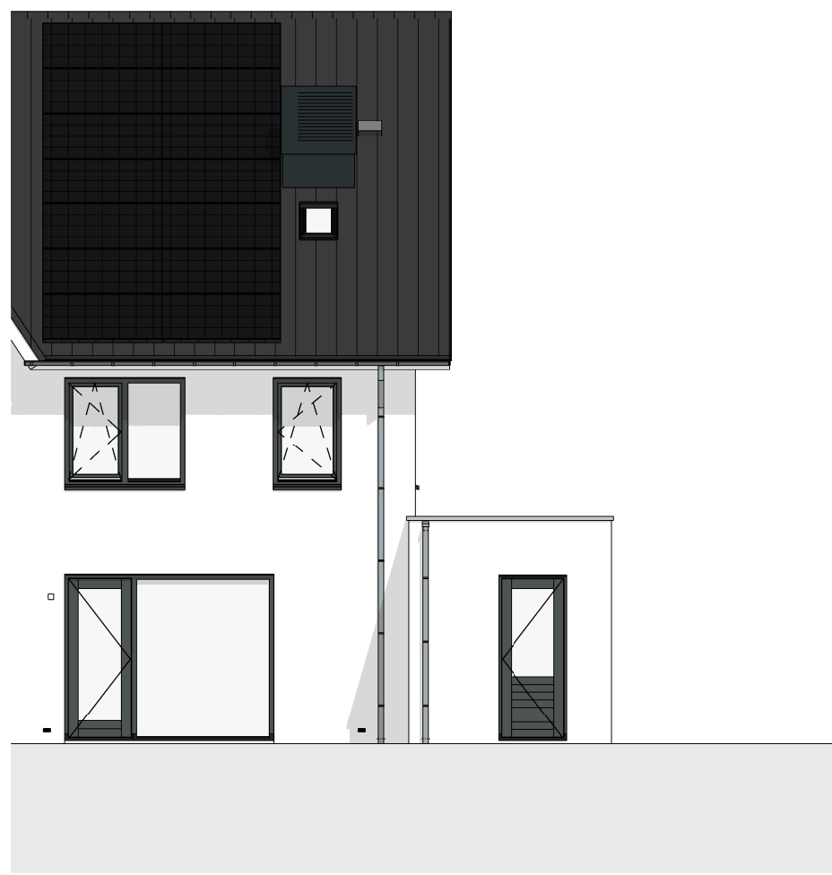
Achtergevel 1 : 100
