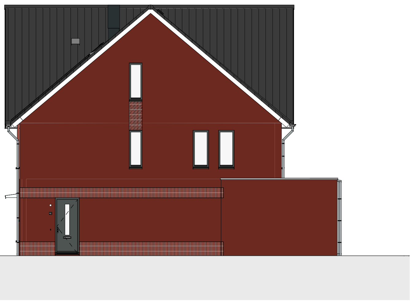
Rechter zijgevel 1 : 100
