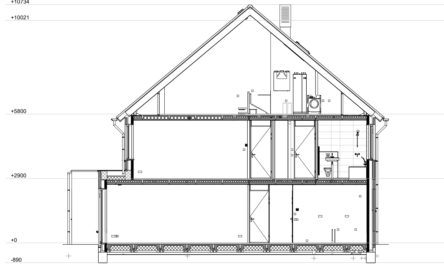
Doorsnede A-A 1 : 100
