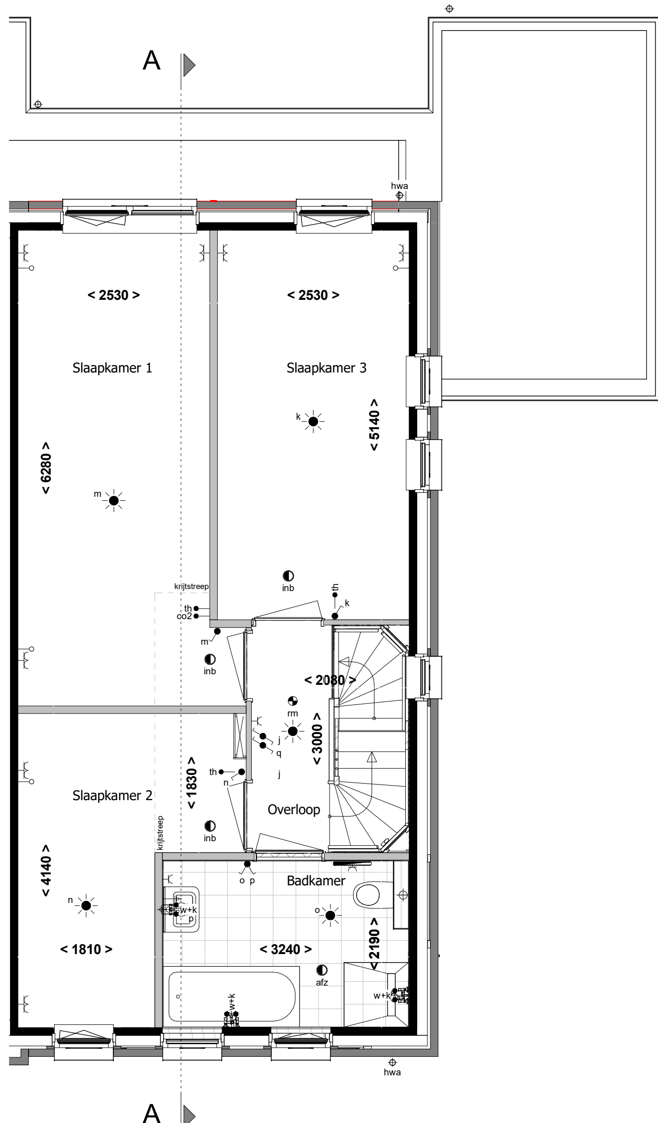
1e verdieping 1 : 50
