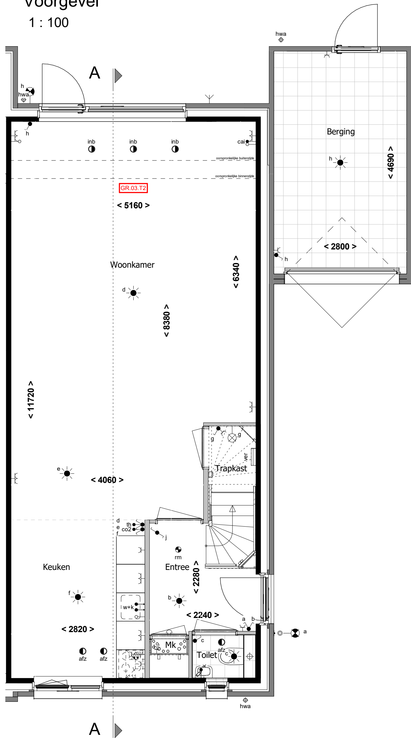
Begane grond 1 : 50
