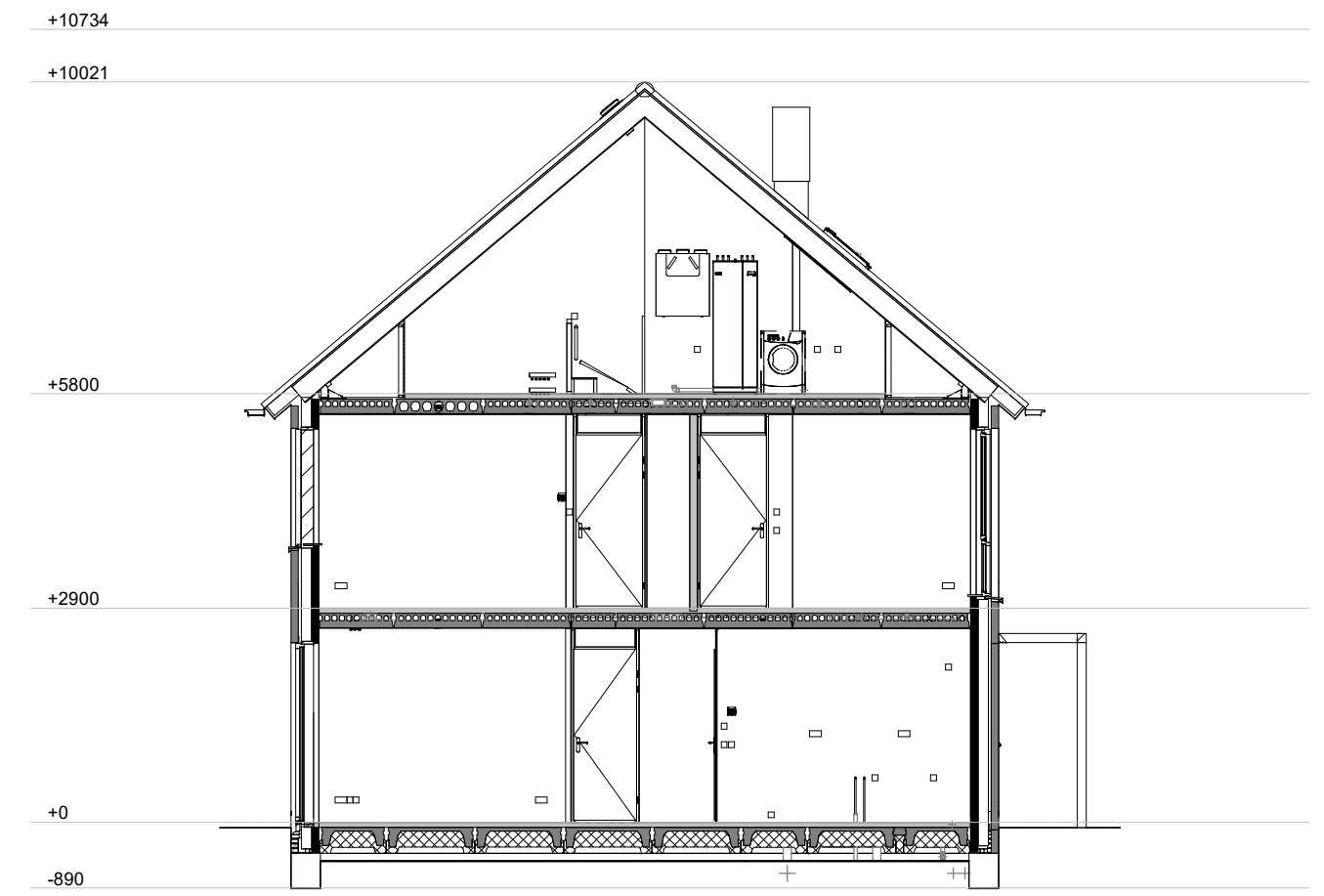
Doorsnede A-A 1 : 100
