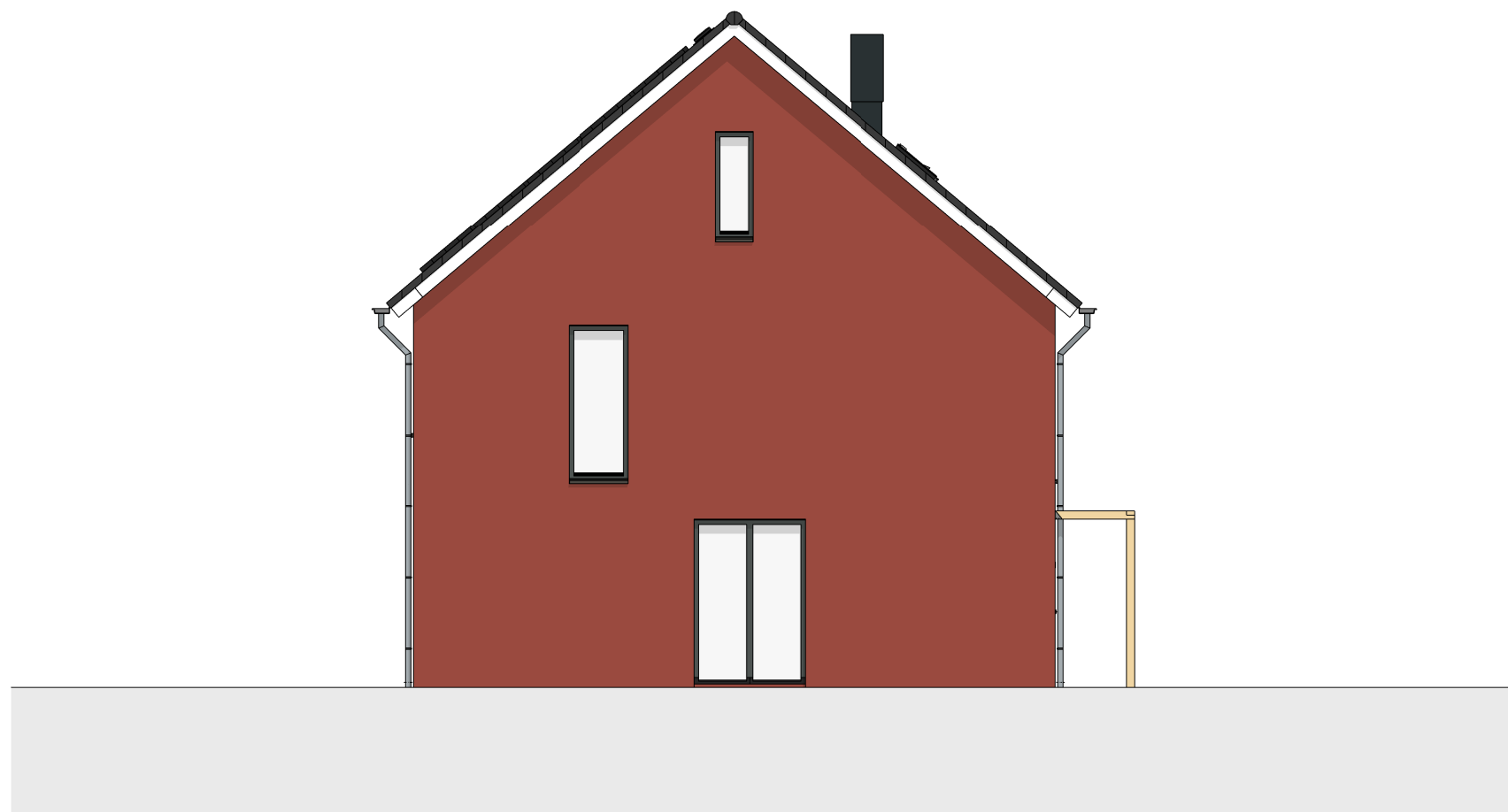
Linker zijgevel 1 : 100
