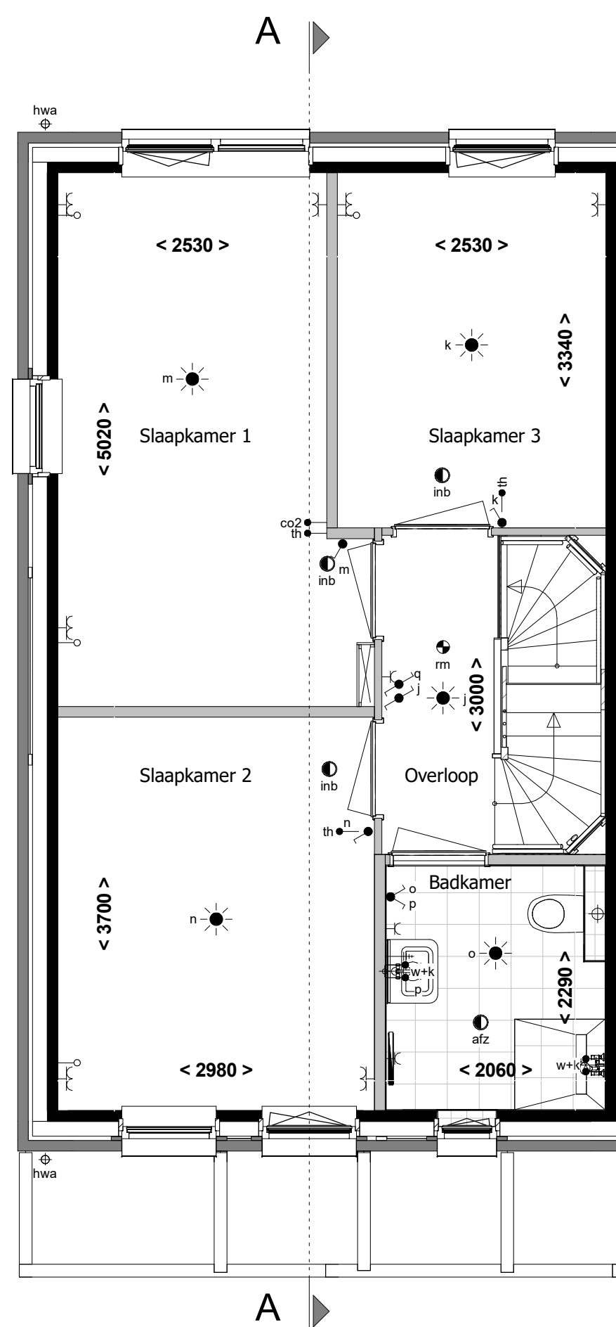
1e verdieping 1 : 50
