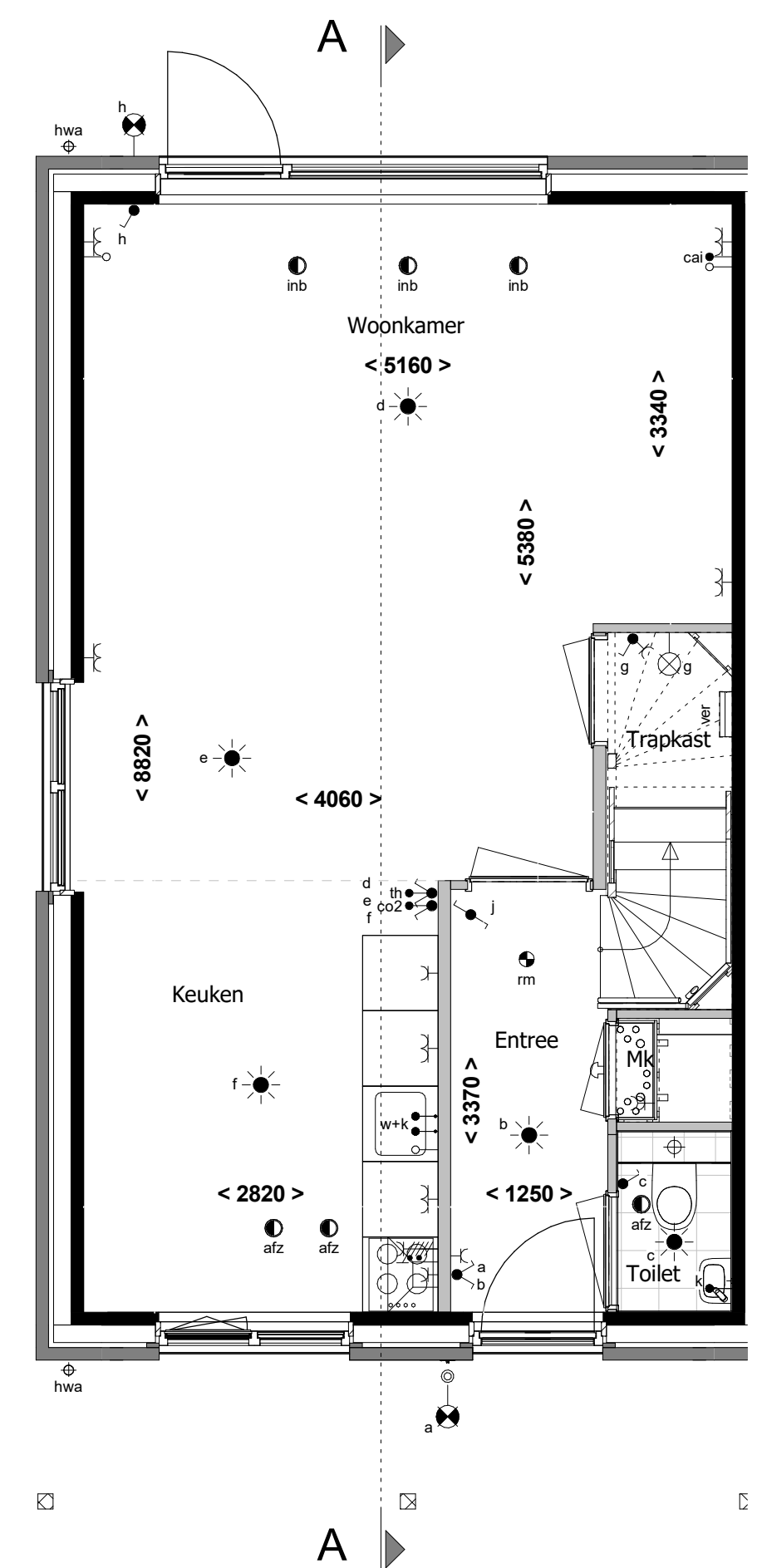
Begane grond 1 : 50
