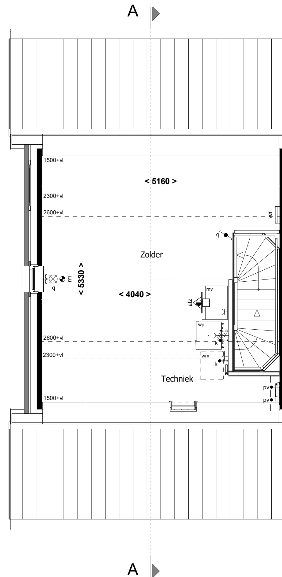
2e verdieping 1 : 50
