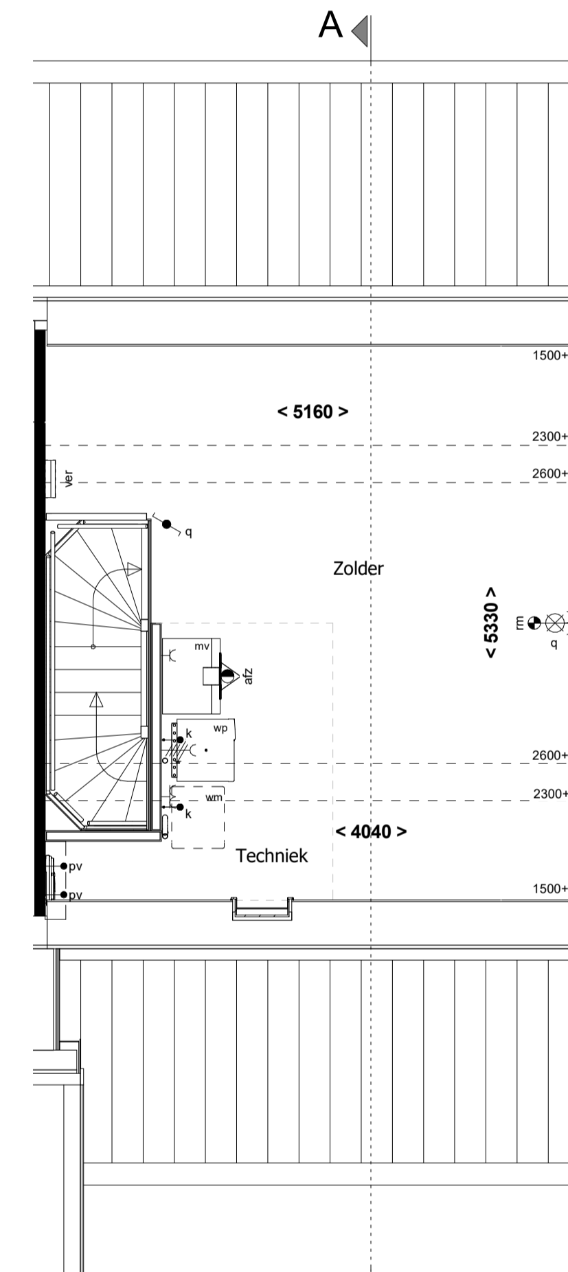
2e verdieping 1 : 50
