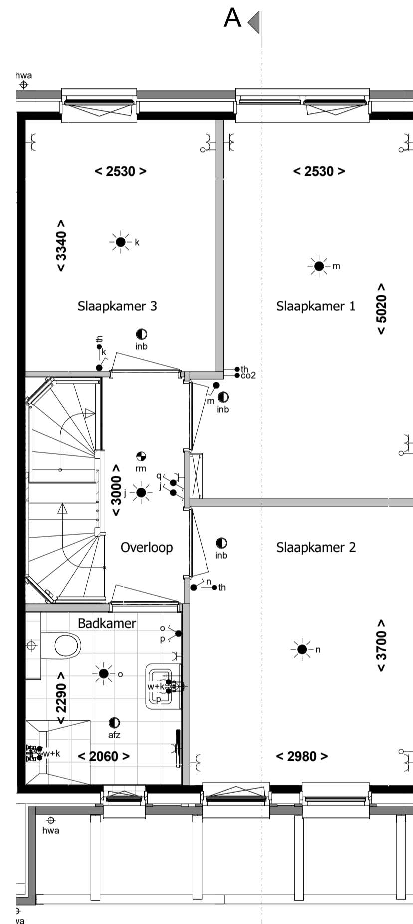
1e verdieping 1 : 50
