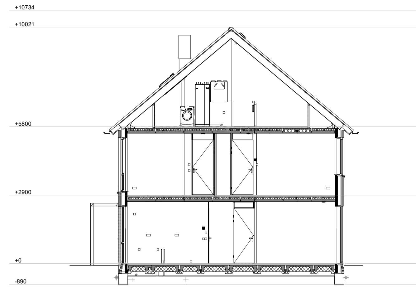
Doorsnede A-A 1 : 100
