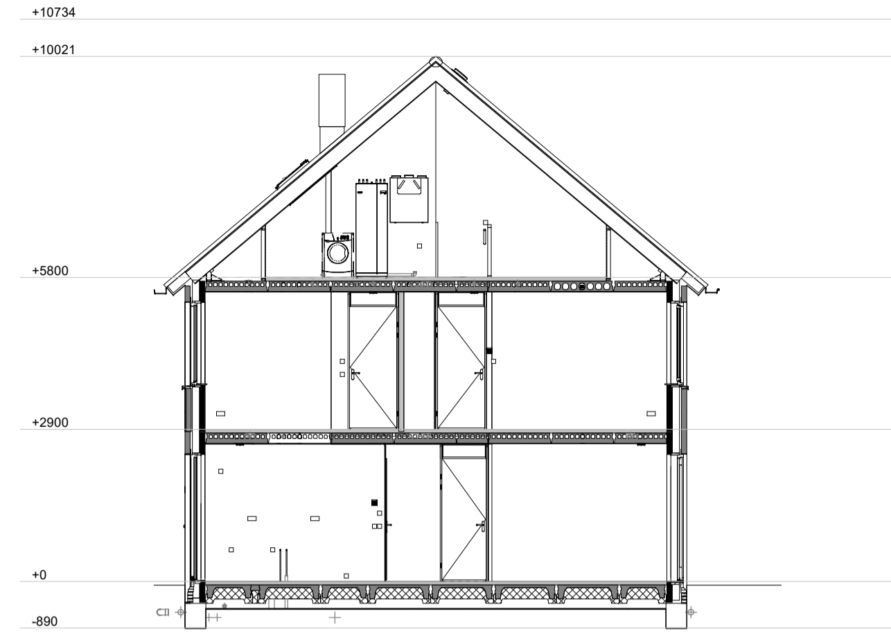
Doorsnede A-A 1 : 100
