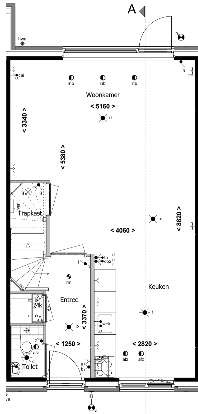
Begane grond 1 : 50
