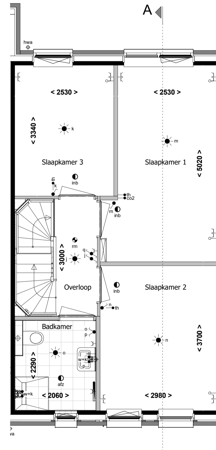
1e verdieping 1 : 50
