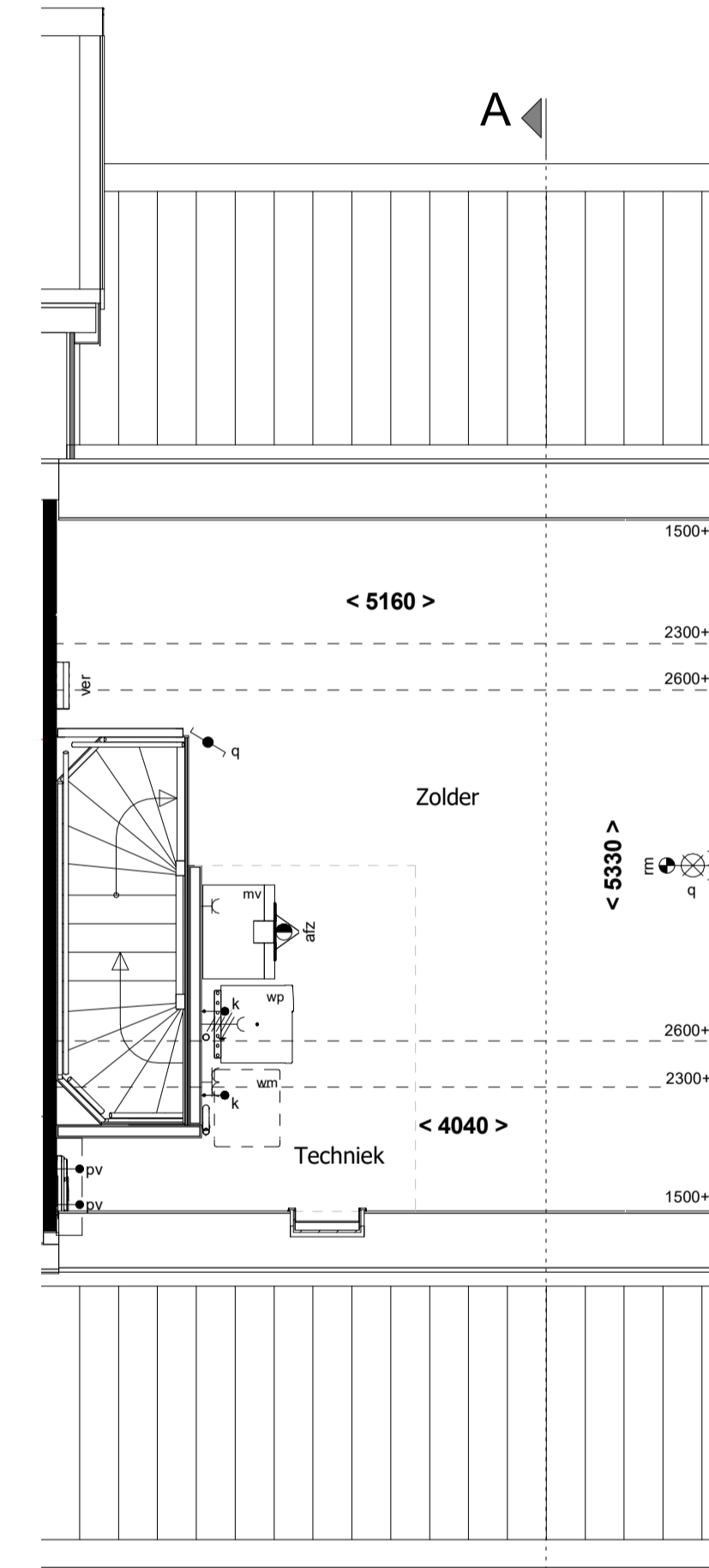
2e verdieping 1 : 50
