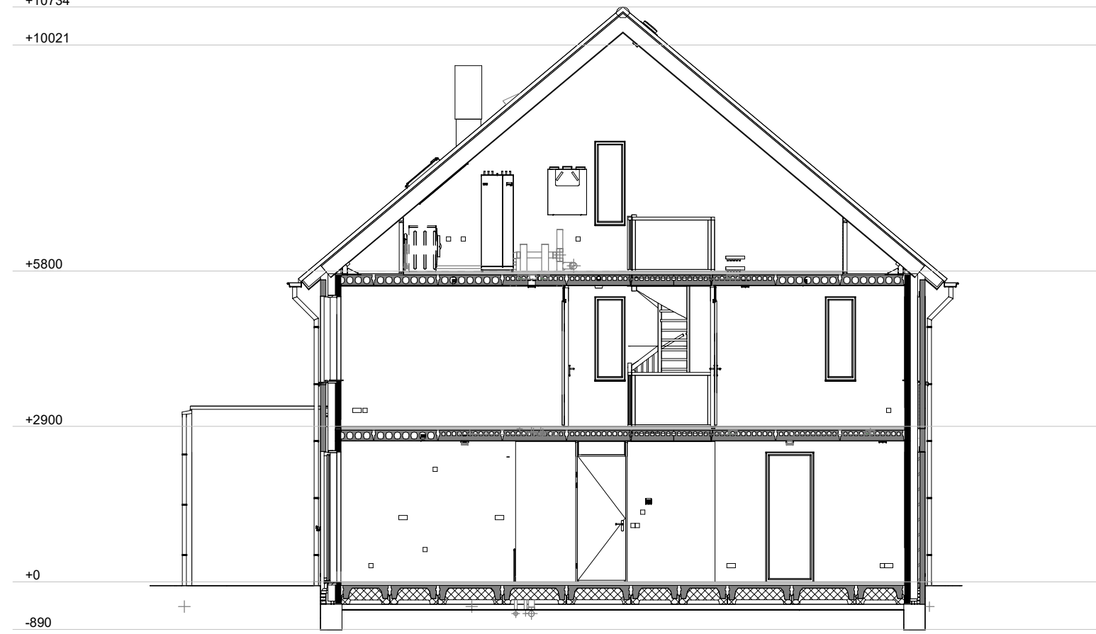
Doorsnede A-A 1 : 100
