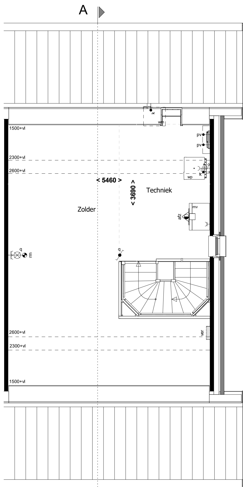
2e verdieping A 1 : 50
