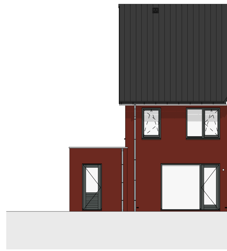
Achtergevel 1 : 100
