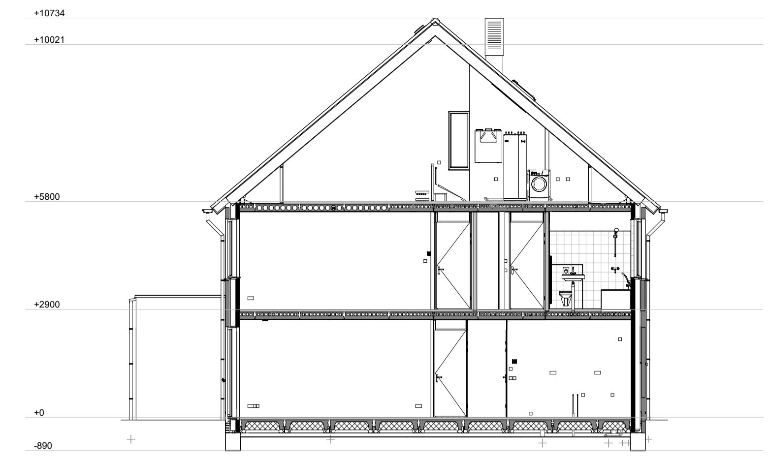
Doorsnede A-A 1 : 100
