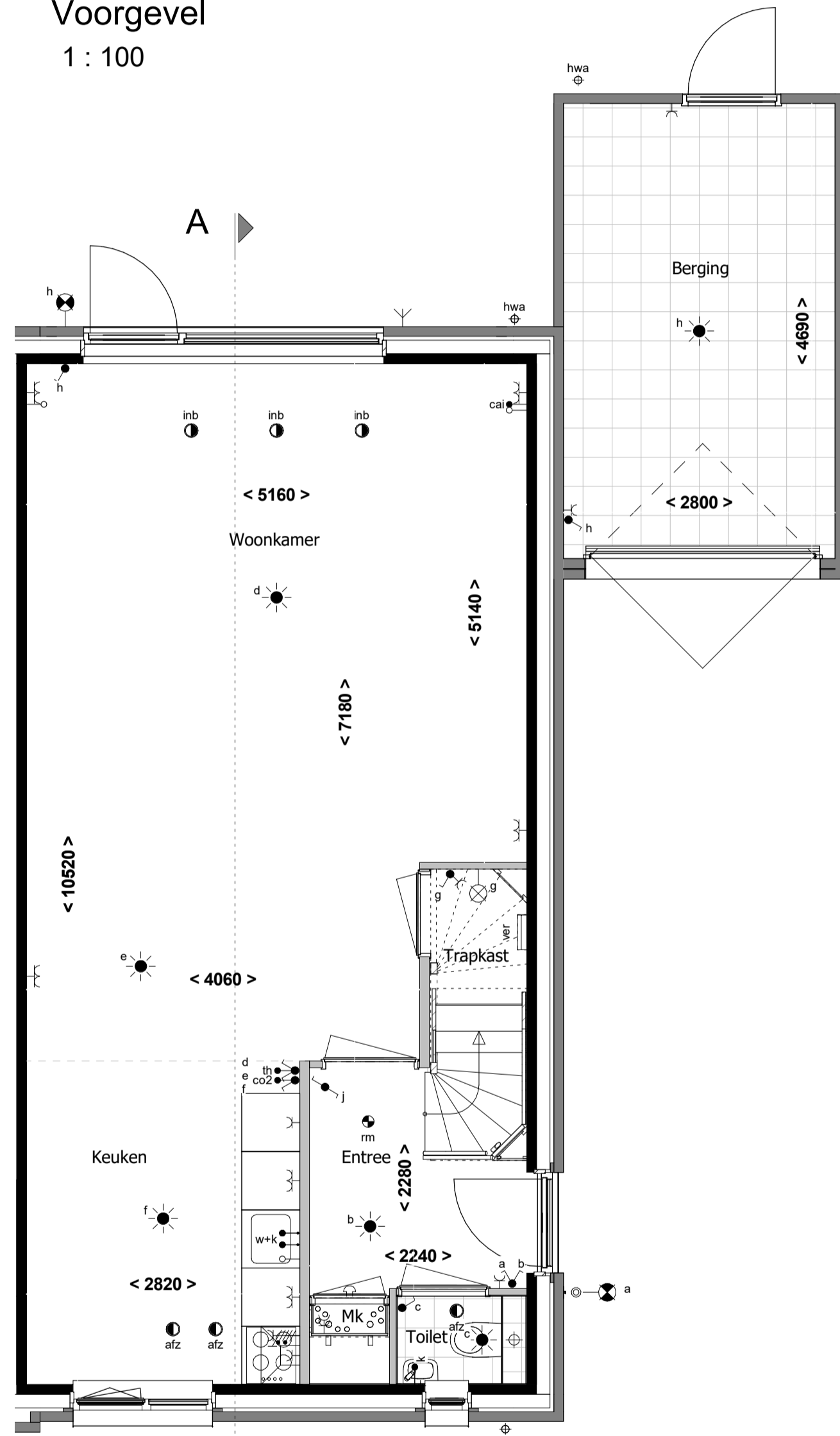
Begane grond 1 : 50
