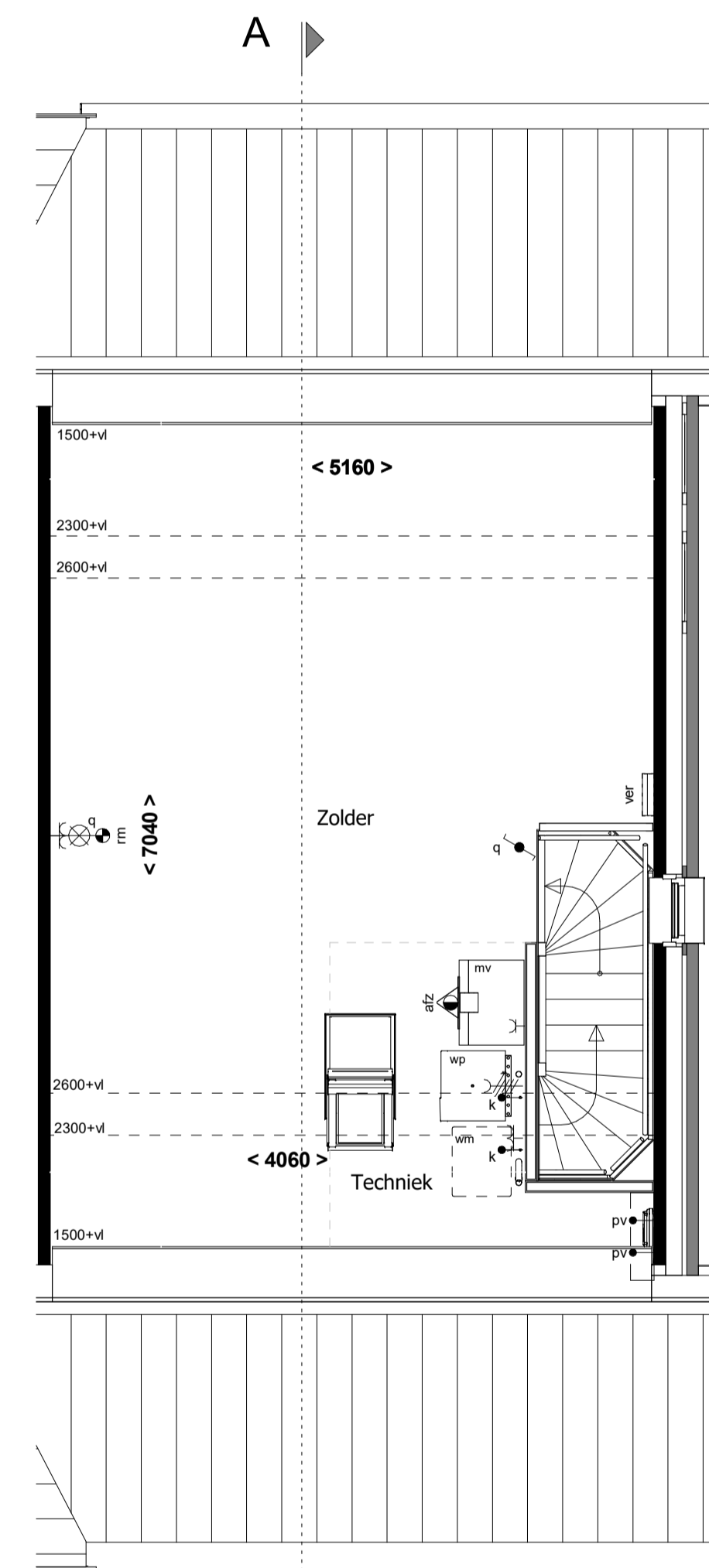
2e verdieping 1 : 50
