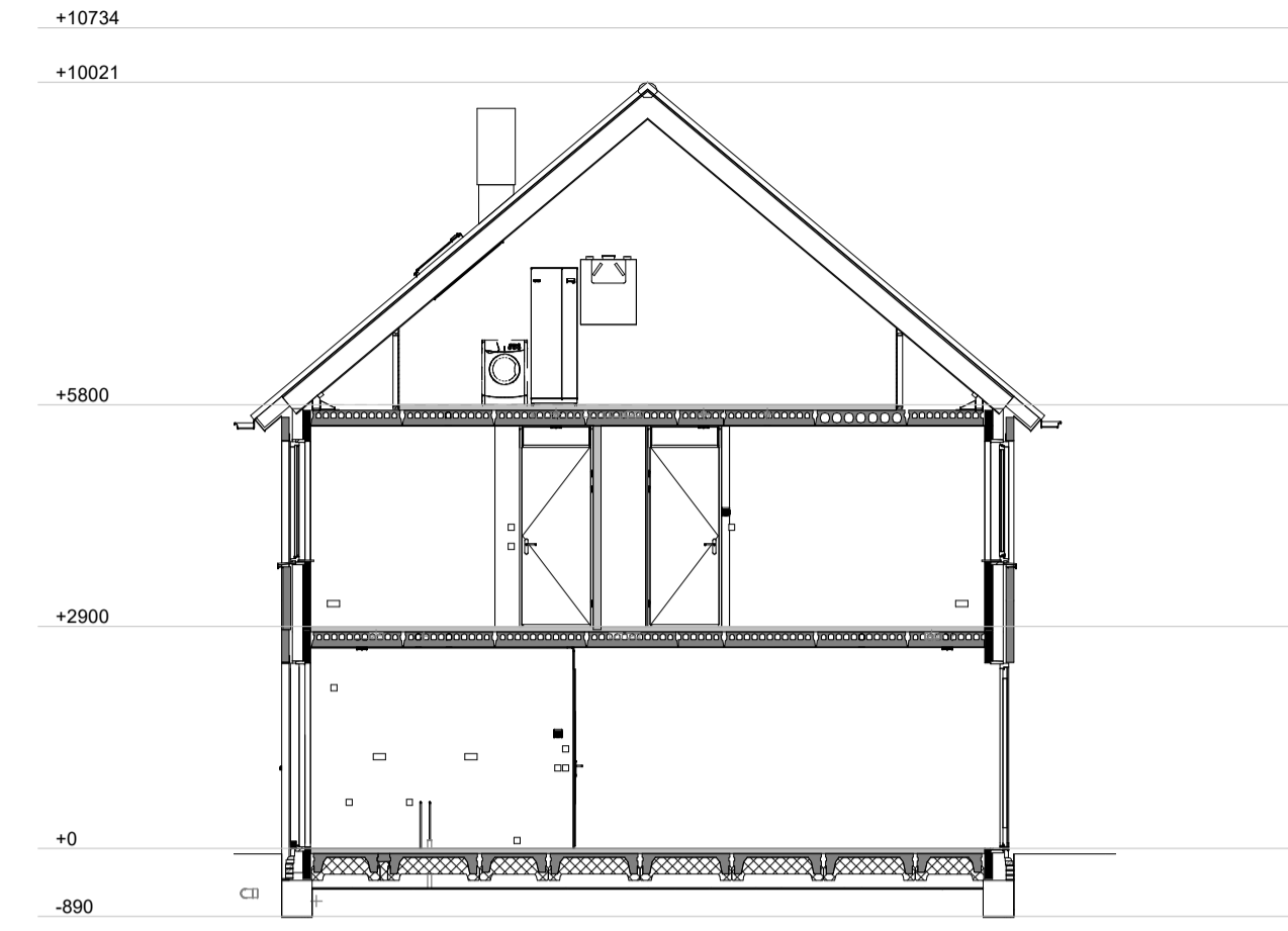
Doorsnede A-A 1 : 100
