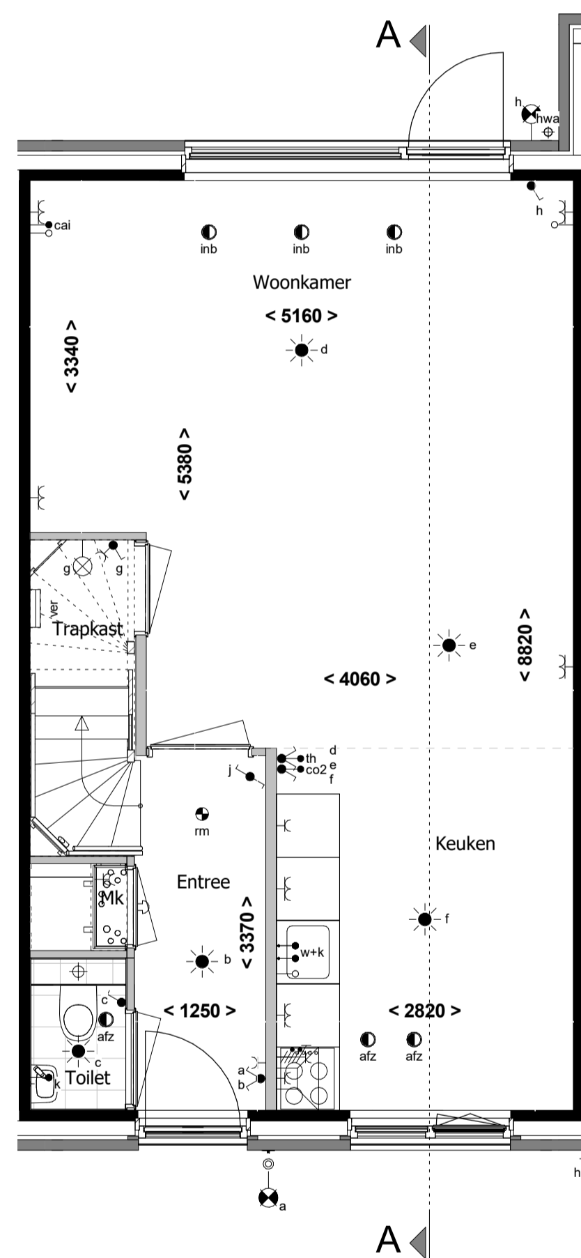
Begane grond 1 : 50
