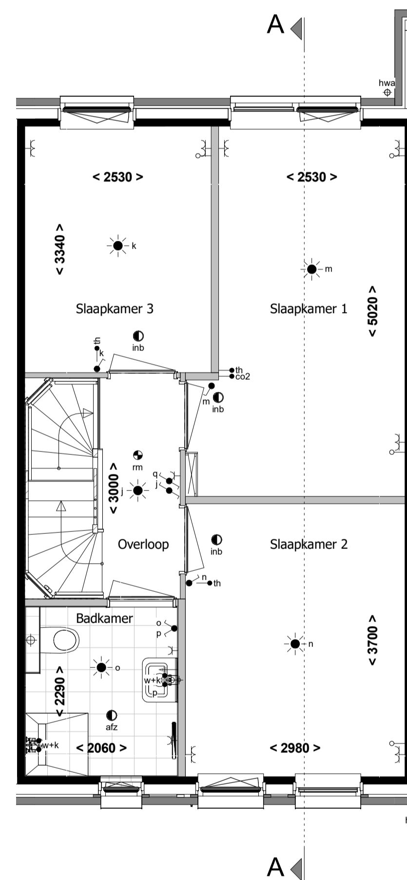
1e verdieping 1 : 50
