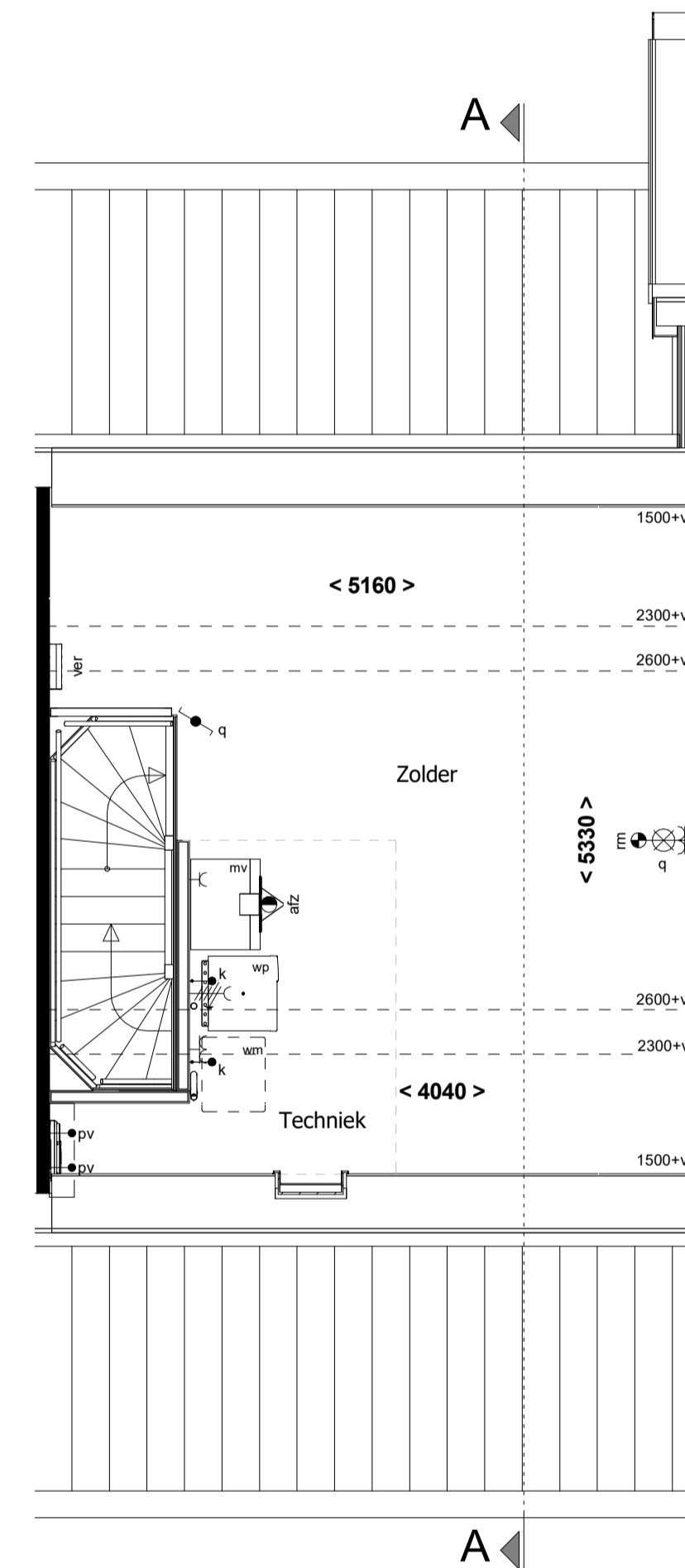
2e verdieping 1 : 50
