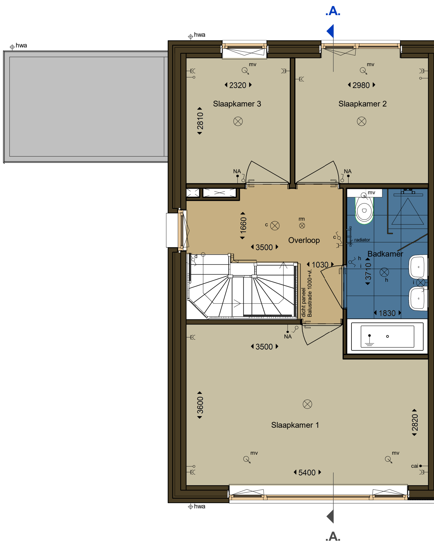
Type A Bnr. 2/4/6/8/10/12/14/16/18/20 eerste verdieping 1:50
